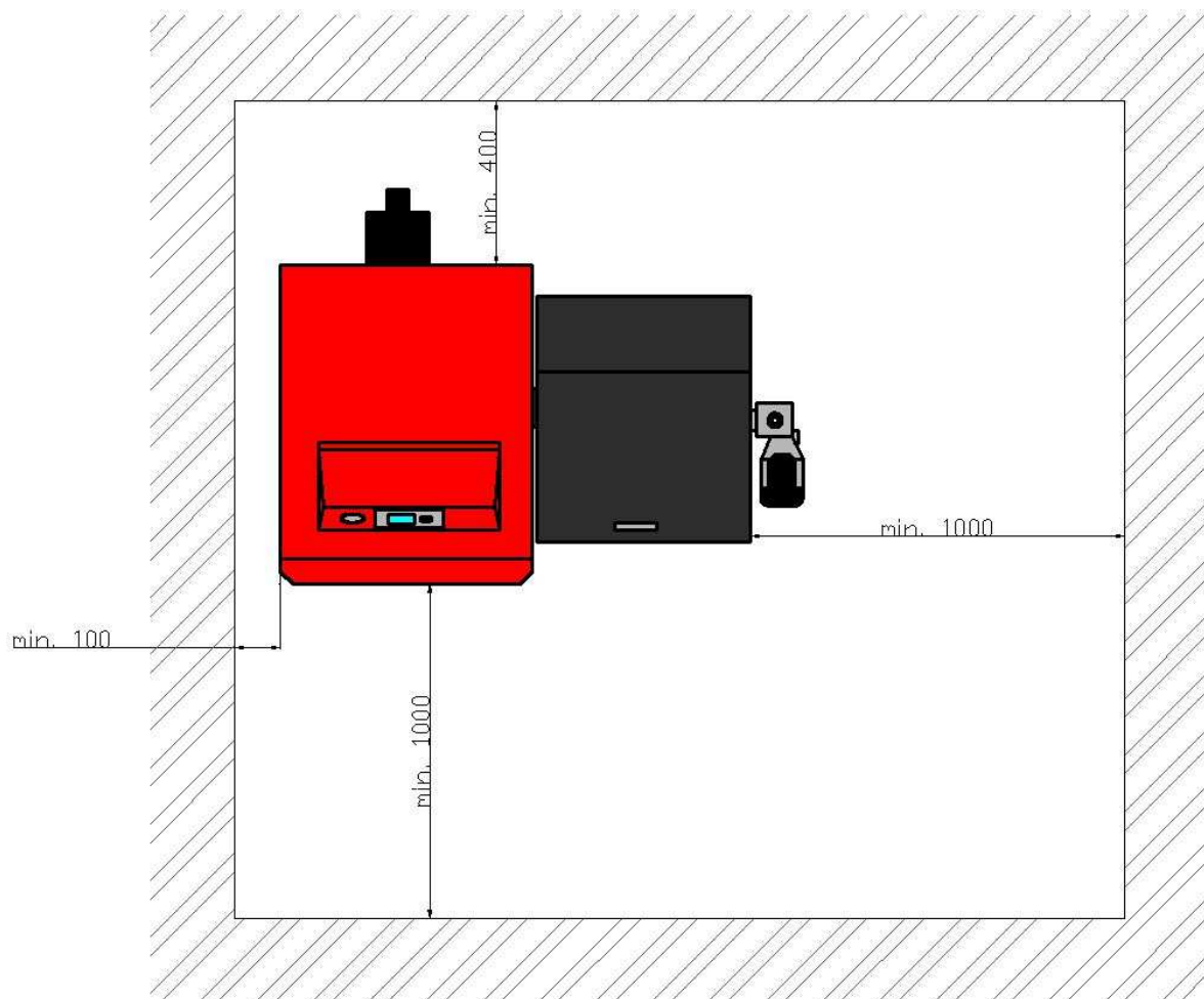
Obr. č. 2 Umístění kotle
