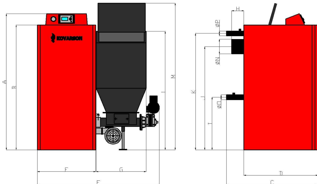
Obr. č. 1 Hlavní rozměry kotle (pravé provedení)
