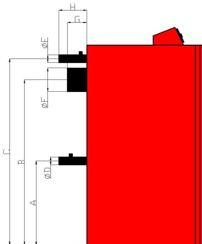
Obr. č. 12 Připojovací rozměry kotlů
